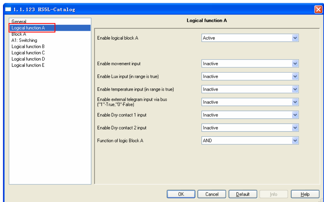
Fig2: “Logical function A” parameter windows
